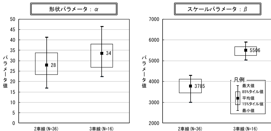
図 3-1-8 ワイブル分布のパラメータ推定結果 7)
