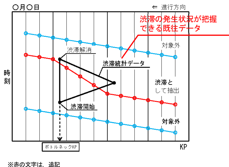
図 2-4-3 渋滞時における ETC2.0 プローブ情報（走行履歴データ）の抽出方法 42)
