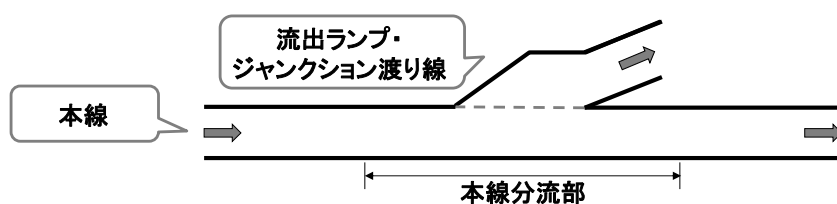
図 2-2-8 本線分流部の道路構造と用語の説明
