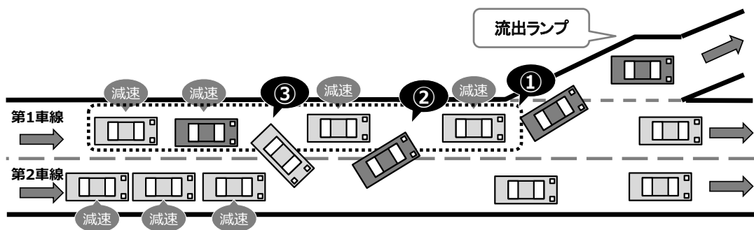
図 2-2-10 本線分流部の渋滞発生メカニズム
