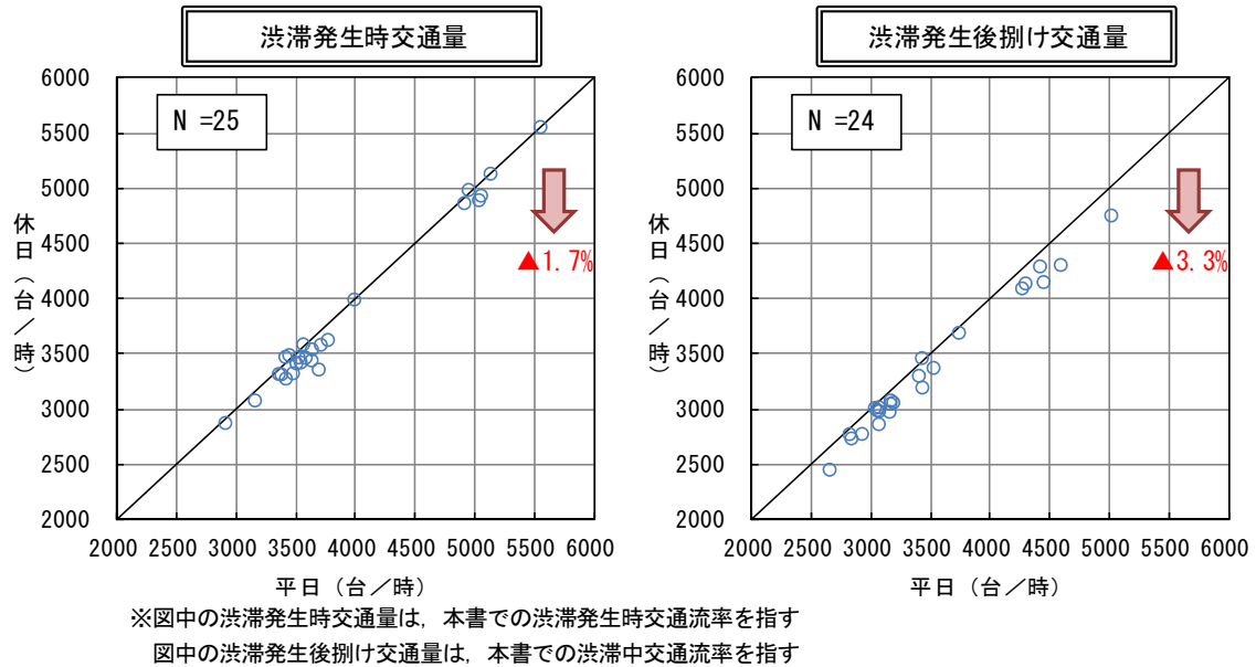
図 3-2-5 曜日別の交通容量比較結果（全時間帯・無降雨） 7)
