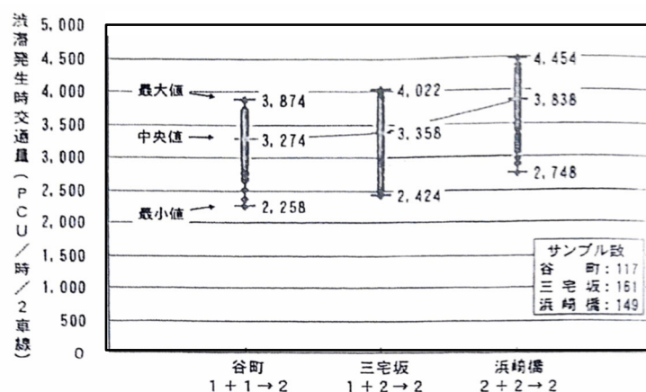
図 3-2-8 合流前後の車線数と渋滞発生時交通流率の関係 53)
