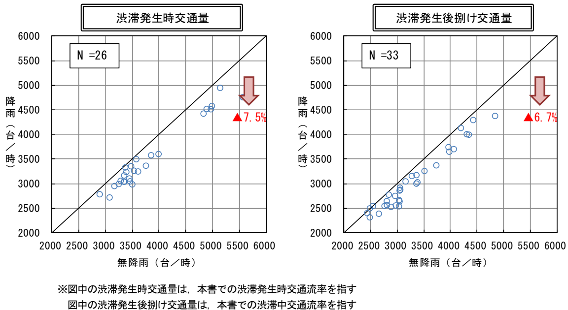
図 3-2-3 無降雨・降雨別の交通容量比較結果 (全時間帯) 7)
