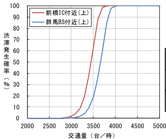
図 3-1-7 関越道（上）の渋滞発生確率分布 7)
