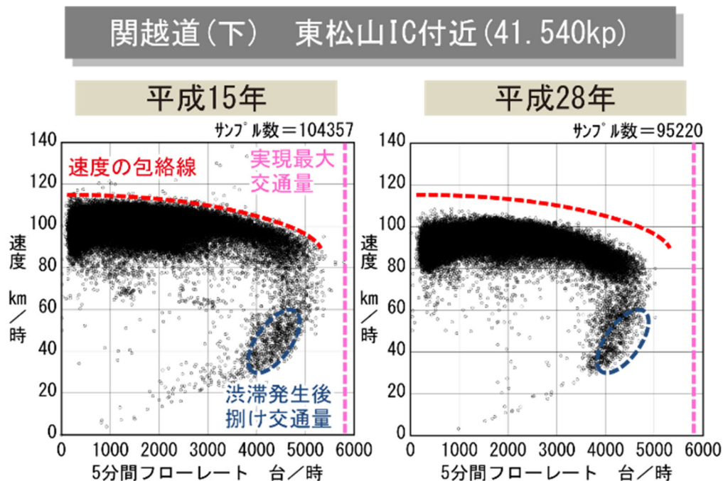
図 3-2-7 QV 図の時点変化例 37)
