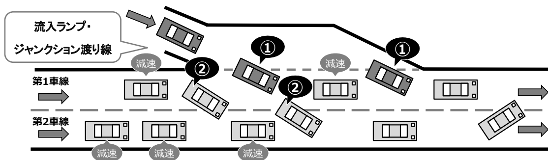
図 2-2-7 本線合流部の渋滞発生メカニズム
