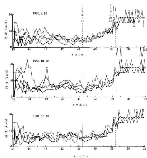
＜地点速度変動図による BN 位置特定例＞
