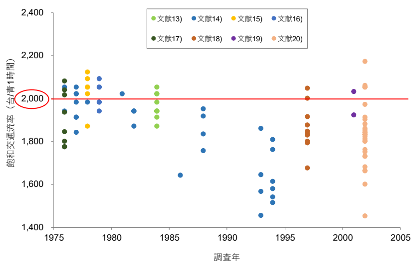
図 4-2-1 既存文献で観測された飽和交通流率 21)
