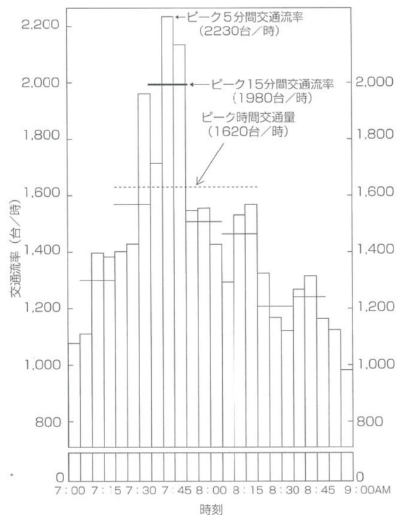
交通流率と時間交通量の関係 15)
