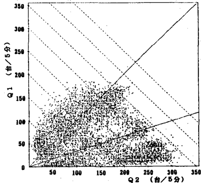
図 3-2-9 流入ランプの交通量と合流前の本線の交通量の関係 56)
