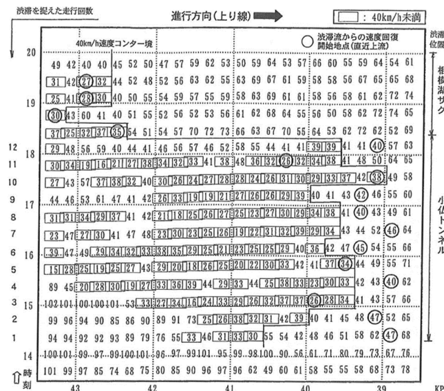
＜速度コンター図による BN 位置特定例＞
