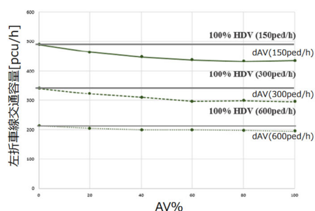
(a) 左折車線の交通容量 31)
