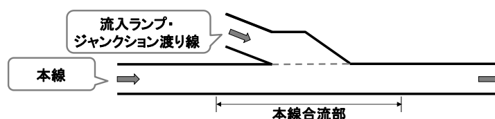
図 2-2-5 本線合流部の道路構造と用語の説明
