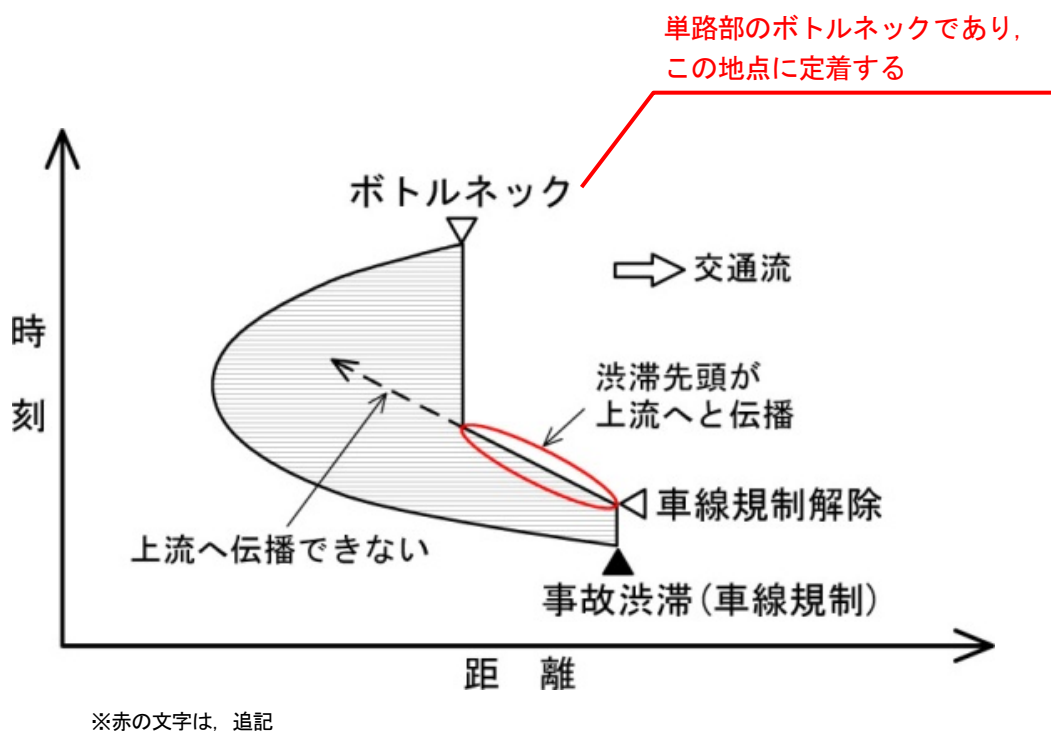
図 2-2-4 典型的な渋滞定着現象の概念図（事故規制解除後の事例） 14)
