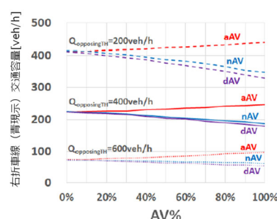
(b) 右折車線の交通容量 32)
