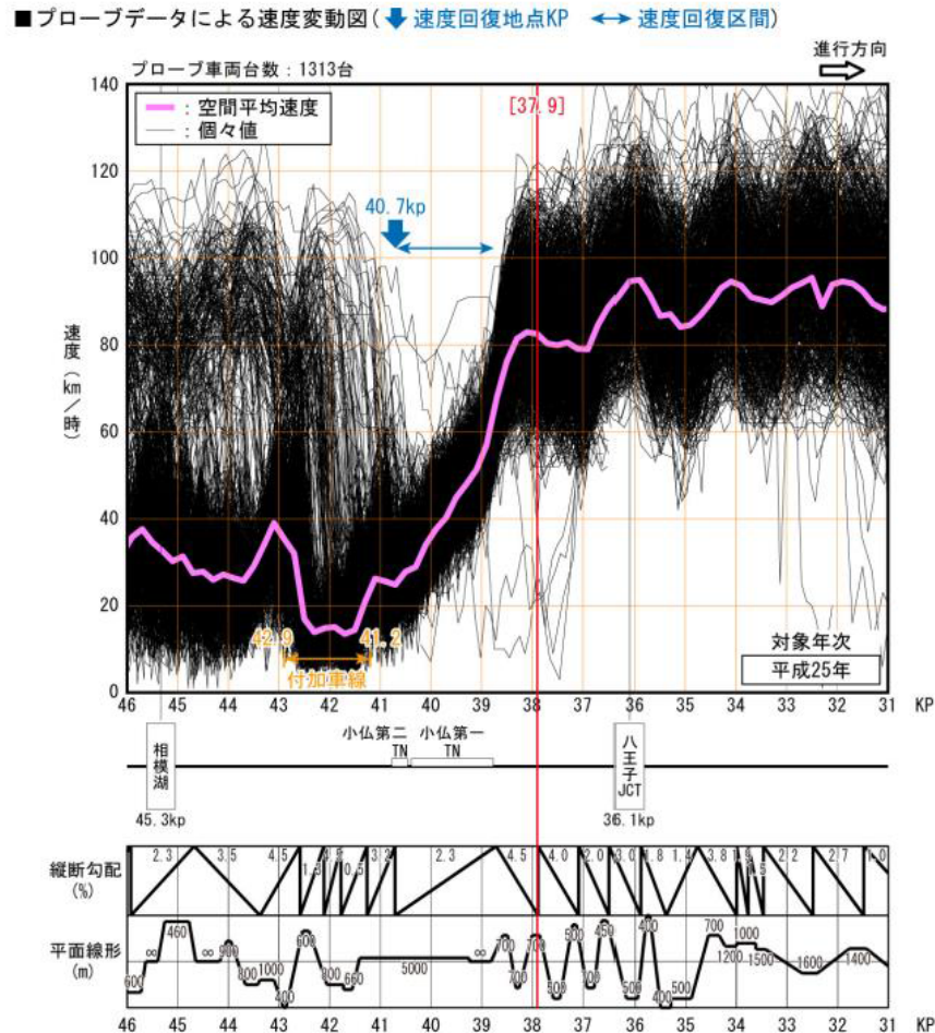
図 2-4-4 渋滞時における ETC2.0 プローブ情報の速度プロファイル例 42)
