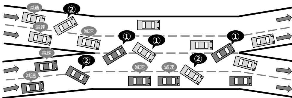
図 2-2-11 織り込み区間の渋滞発生メカニズム
