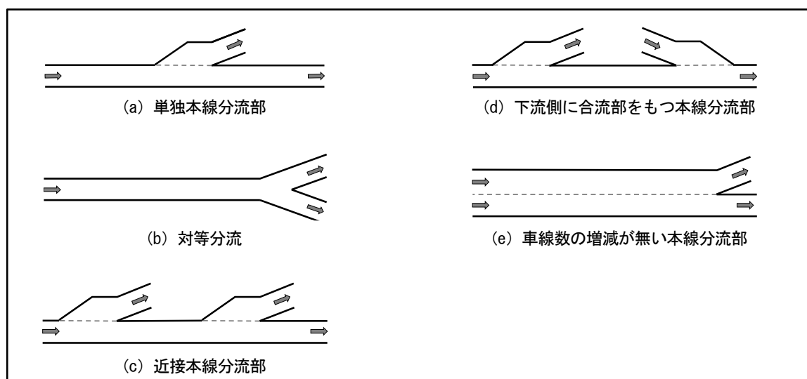
図 2-2-9 本線分流部の種類
