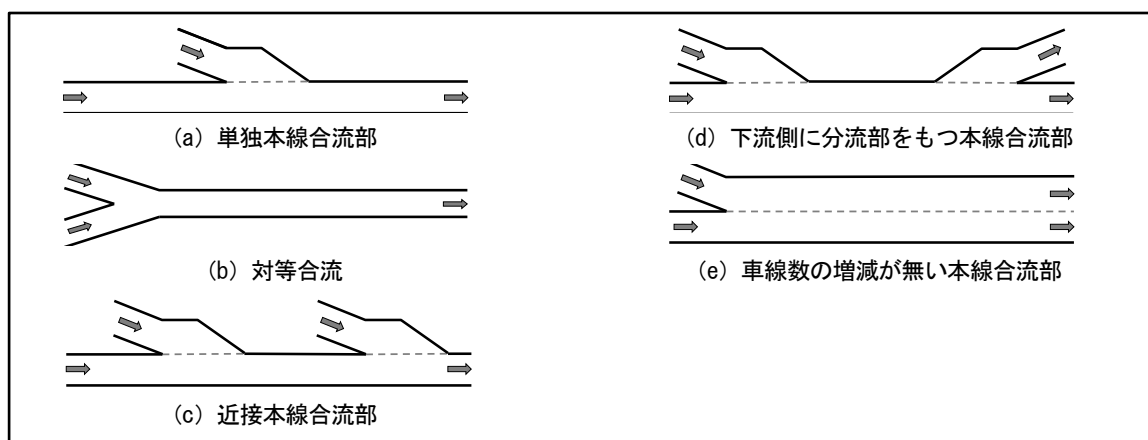
図 2-2-6 本線合流部の分類
