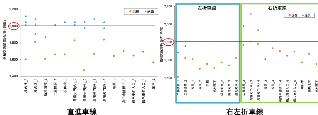
図 4-2-2 過去と現在の飽和交通流率の観測結果 21)
